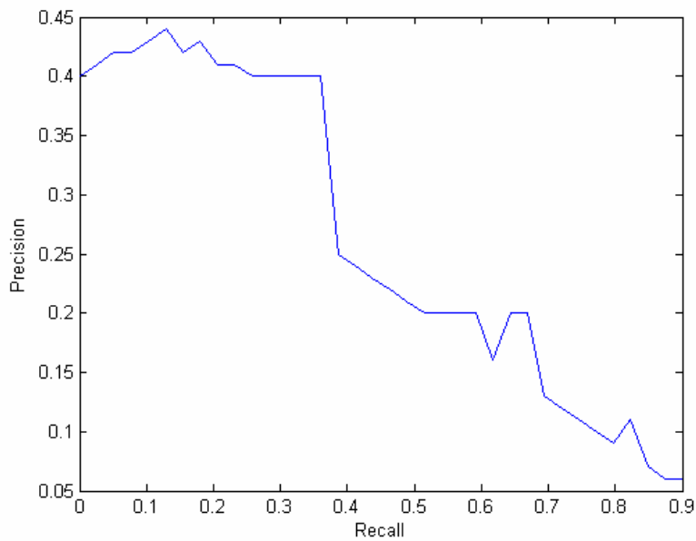
Fig.3 the average recall-precision curve of the SOM
